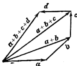
Рисунок 83. Правило многоугольника
