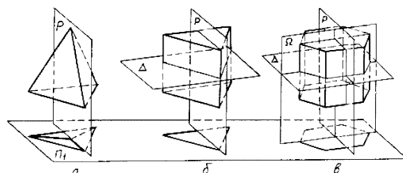
Рисунок 40. Плоскости симметрии
