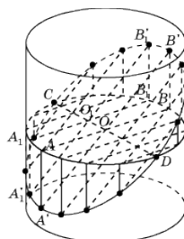
Рисунок 61. Сечение цилиндра
