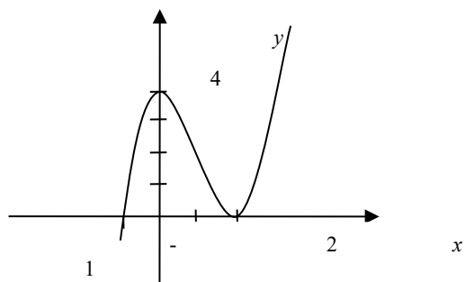
Рисунок 23. График функции y=(x+1) \cdot (x-2)^2
