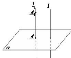
Рисунок 43. Ортогональное проектирование
