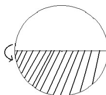
Рисунок 65. Сфера
