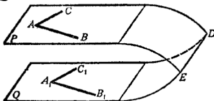
Рисунок 37. Параллельные плоскости
